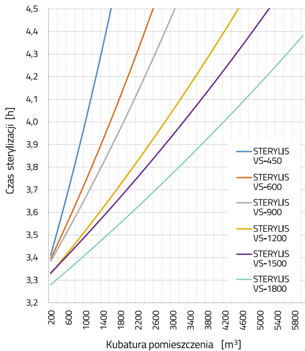
Wykres czasu sterylizacji ozonem w zależności od kubatury pomieszczenia sterylizowanego
